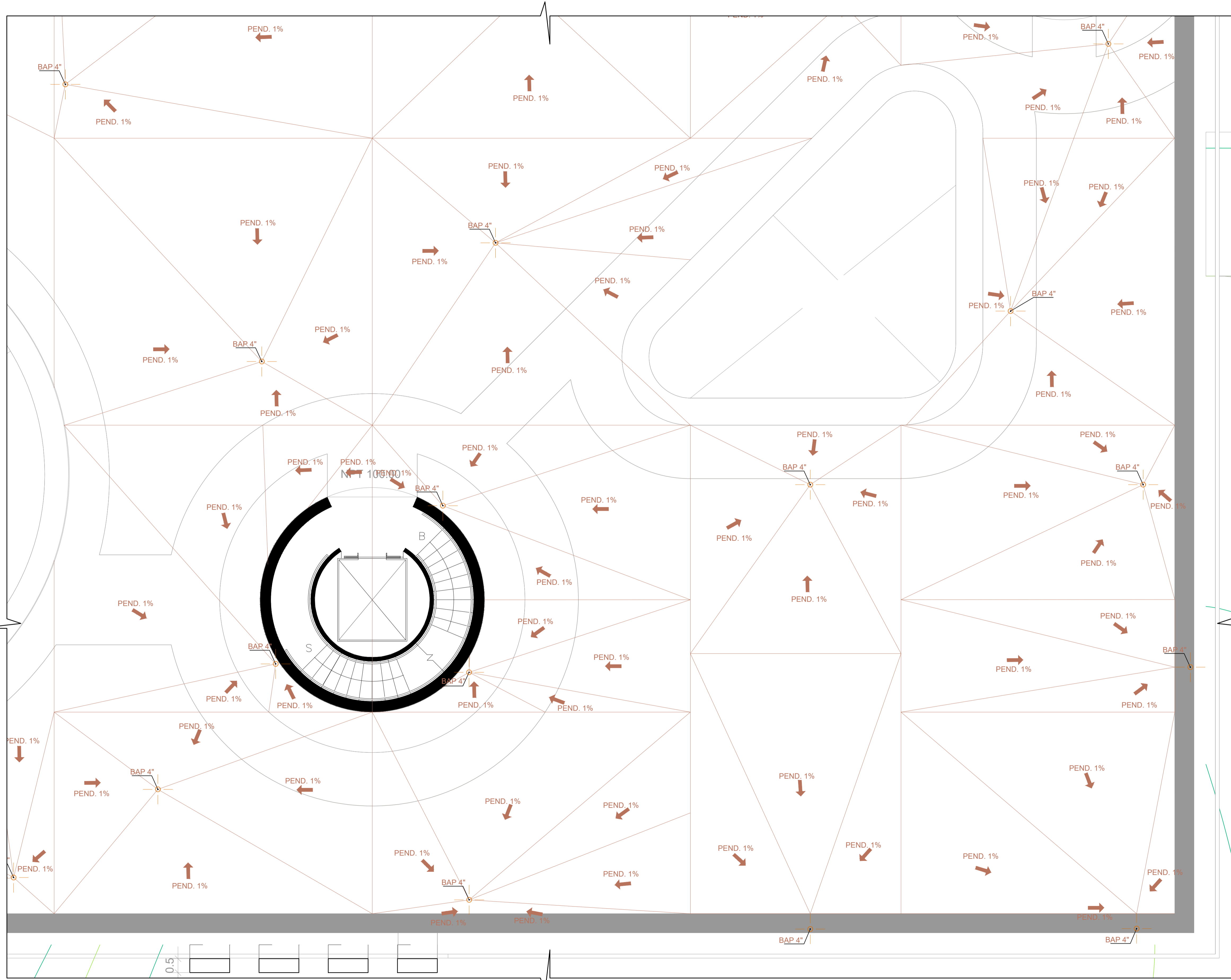
AMPLIACIÓN # 1 DRENAJES PLUVIALES ESCALA 1: 50
